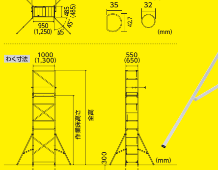
作業床寸法(mm) 485×1,250
